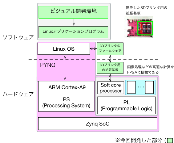
図1 FPGA を利用した 3D プリンタの制御システム
